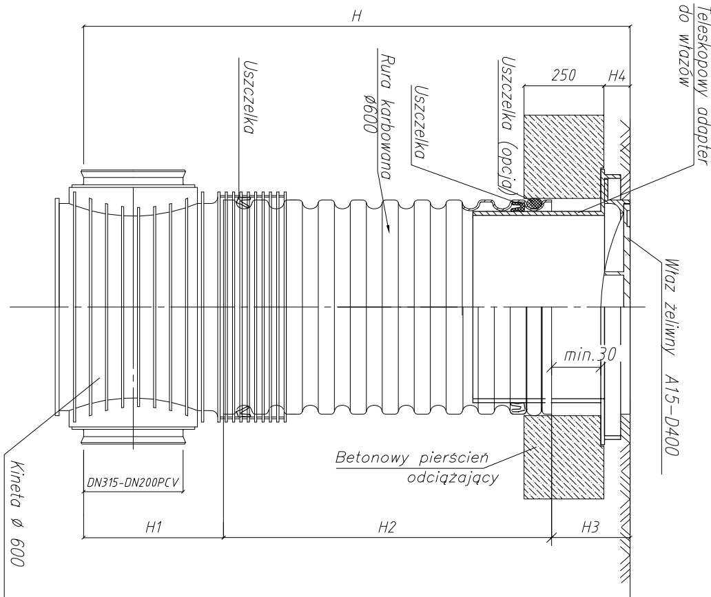
Studzienka inspekcyjna ø600
